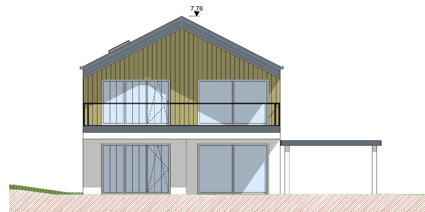
Ansicht SW Haus A M 1:100
