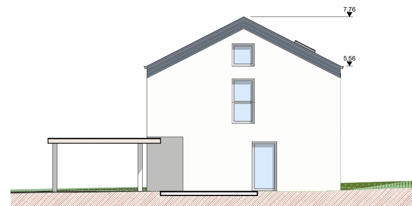
Ansicht NO Haus A M 1:100
