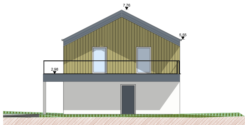
Ansicht SO Haus B M 1:100
