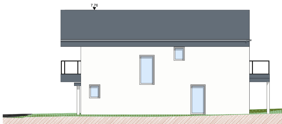
Ansicht NO Haus B M 1:100
