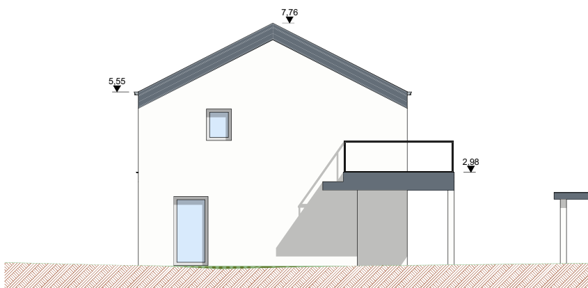
Ansicht NW Haus B M 1:100
