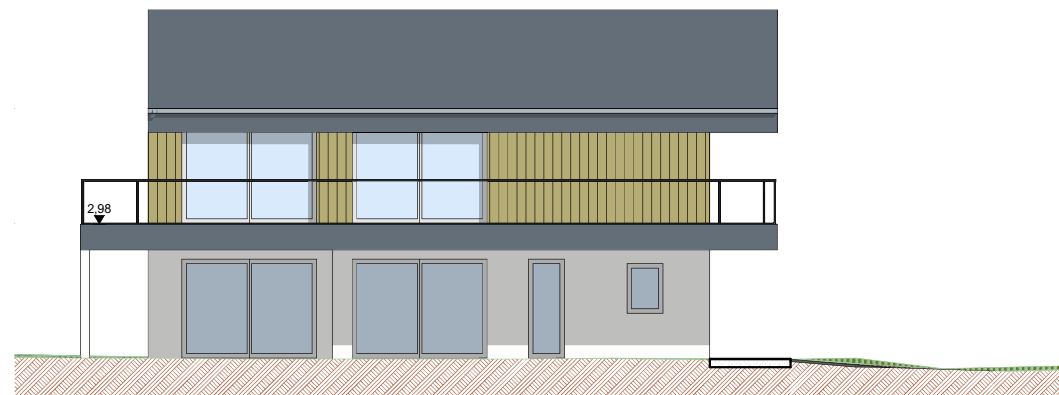
Ansicht SW Haus B M 1:100
