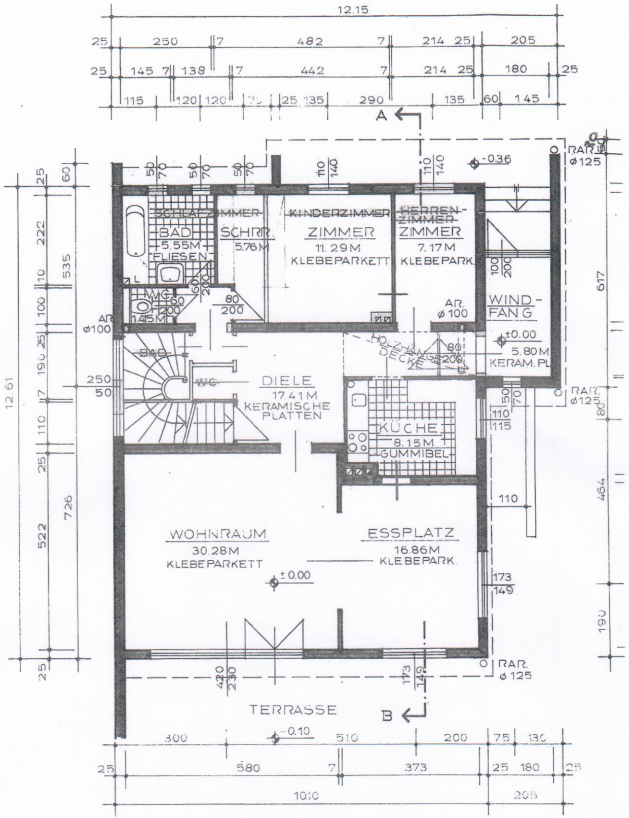
ERDGESCHOSS 44
