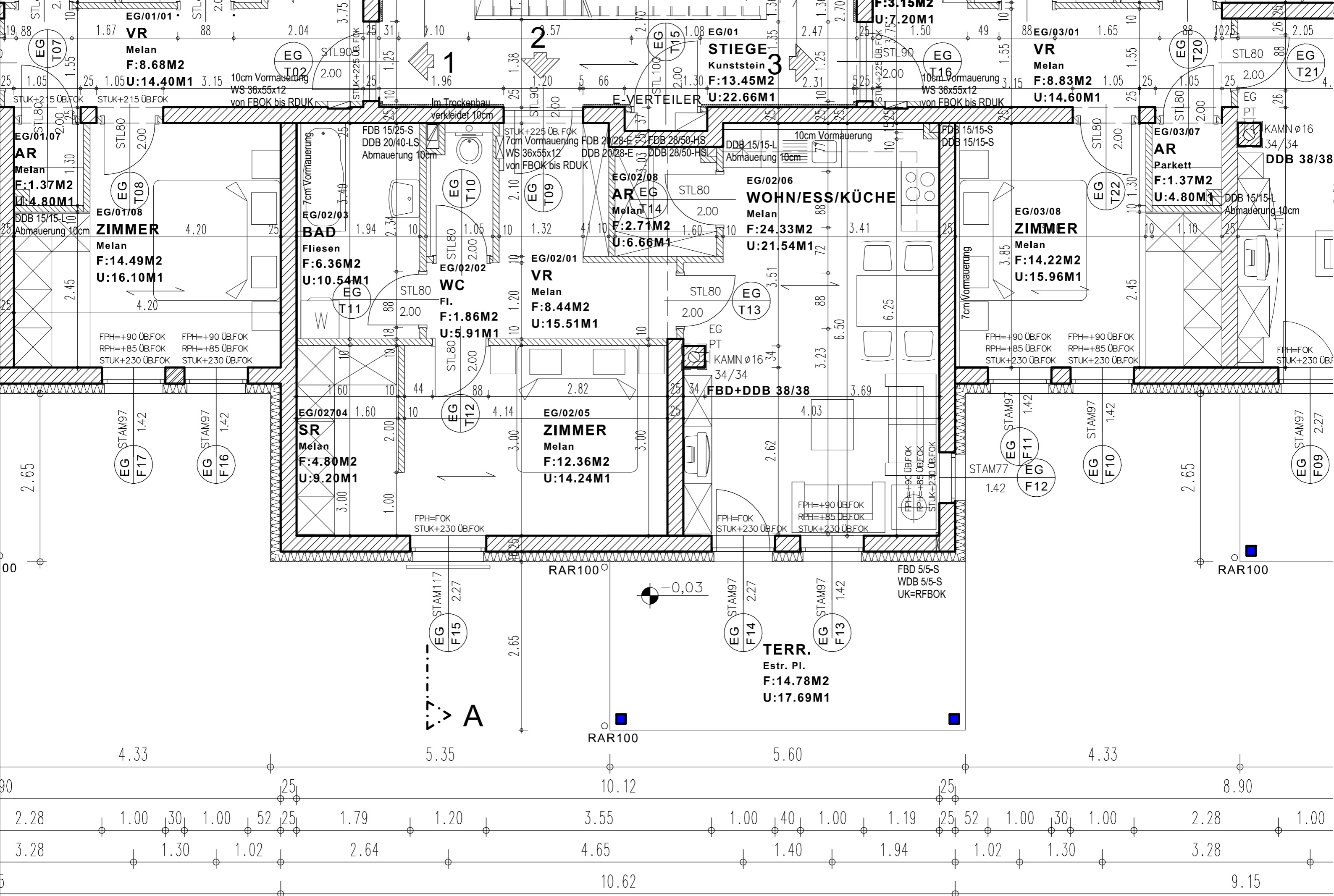
GRUNDRISS ERDGESCHOSS - TOP 2
