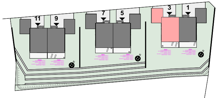
Übersicht M 1:1000
