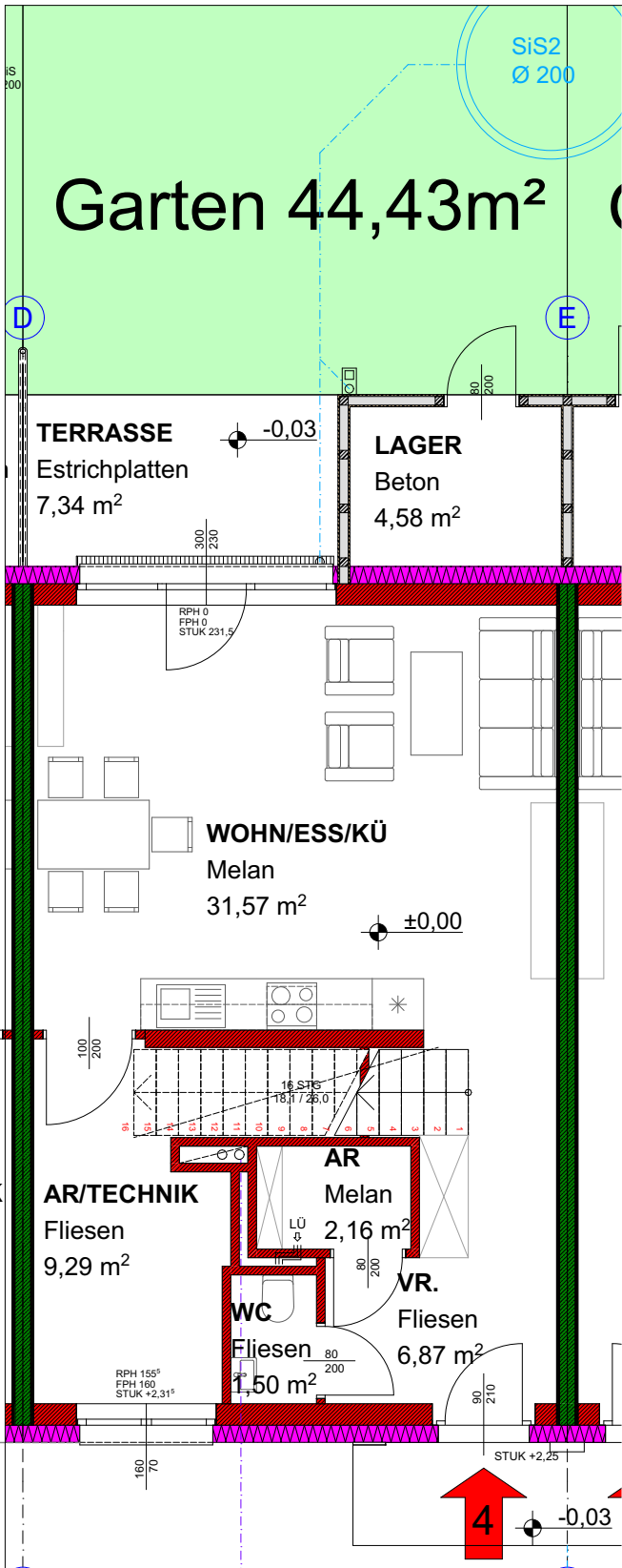
ERDGESCHOSS
