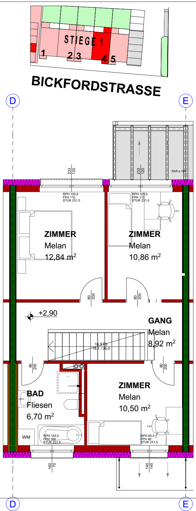
OBERGESCHOSS
