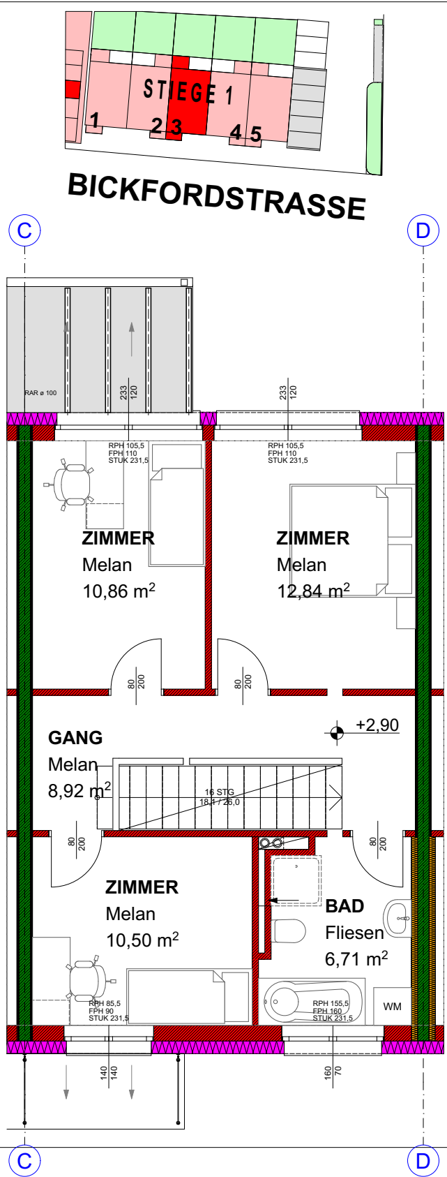
OBERGESCHOSS
