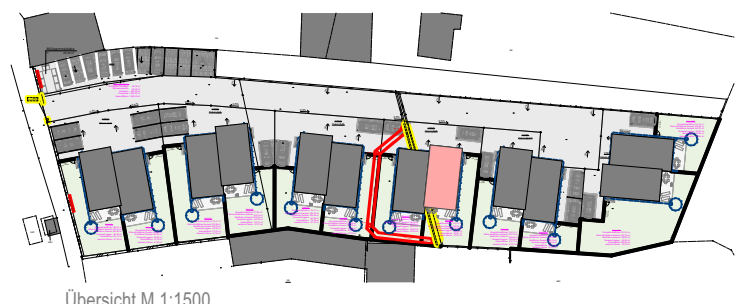
Übersicht M 1:1500
